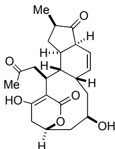
(+)-macquarimicin B (2)
