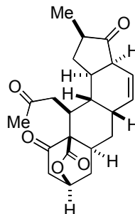
(+)-macquarimicin C (3)
